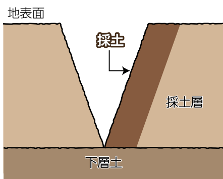
図2 採土方法
